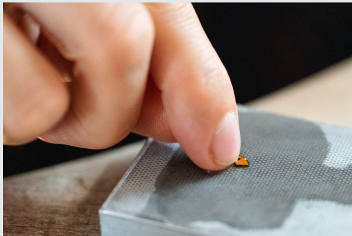
Lapidage de la pièce sur une pièce préalablement humidifiée © Inas HAMAGUCHI
