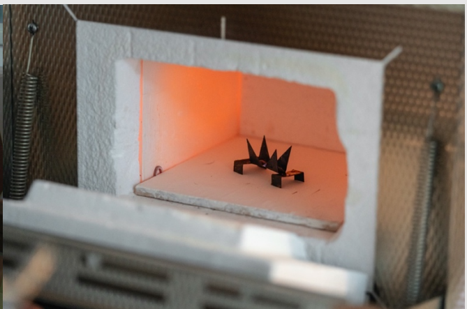
La pièce est enfournée sur un support © Inas HAMAGUCHI
